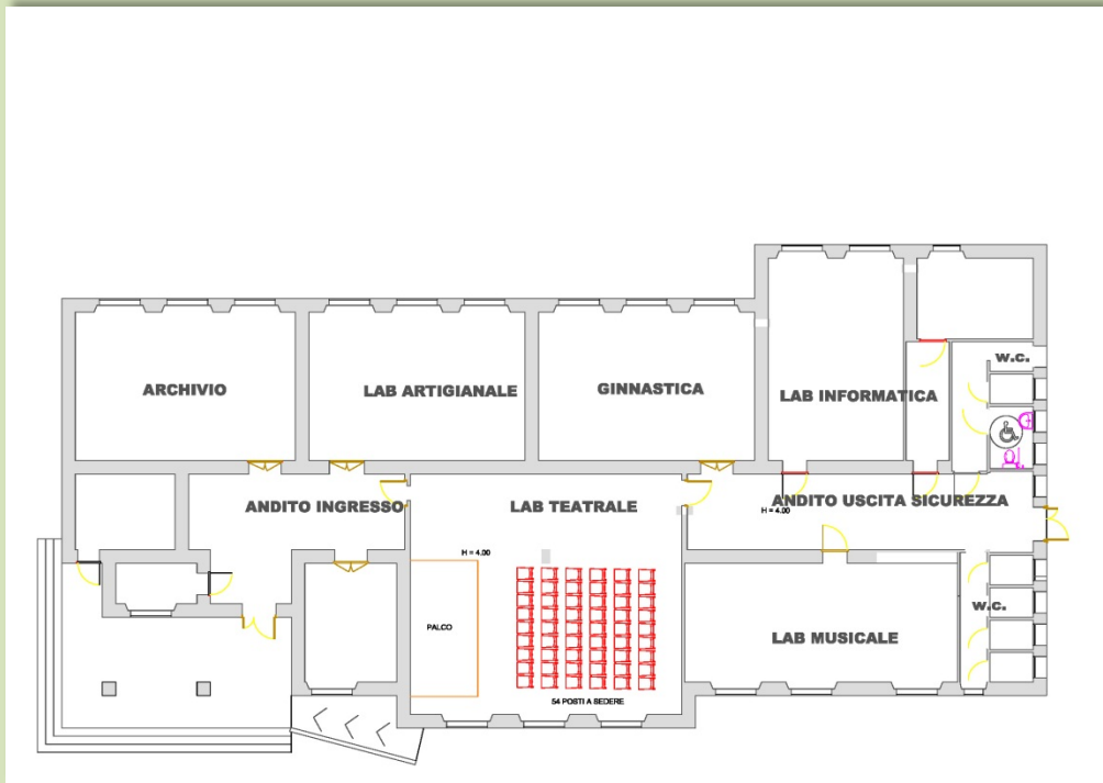
Pianta nuova destinazione d'uso dei locali
